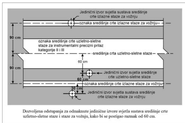
Slika 5-27. Odmaknuti jedinični izvori svjetla sustava svjetala središnje crte uzletno-sletne staze i staze za vožnju
