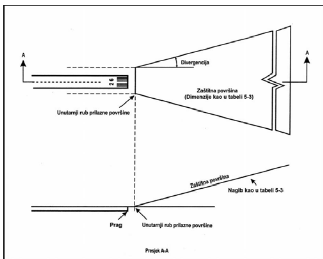
Slika 5-22. Površina slobodna od prepreka za sustave svjetlosnih pokazivača nagiba prilaza
