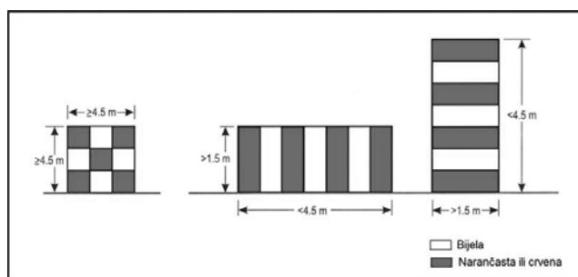
Slika 6-1. Osnovni uzorci označavanja
