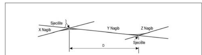
Slika A-2. Profil na središnjoj crti uzletno-sletne staze
