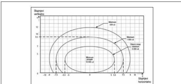
Slika A2.-8. Dijagram izokandela za svjetla na kraju uzletno-sletne staze (crveno svjetlo)
