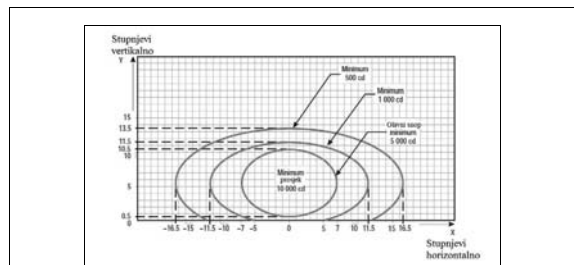
Slika A2-3. Dijagram izokandela za svjetlo praga (zeleno svjetlo)
