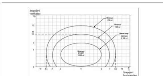
Slika A2-5. Dijagram izokandela za svjetlo područja dodira s kolnikom (bijelo svjetlo)
