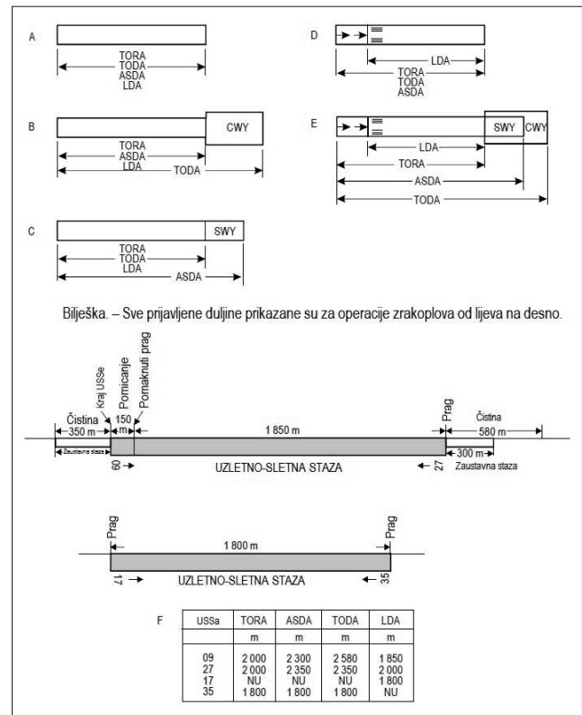
Slika A-1. Prikaz prijavljenih duljina
