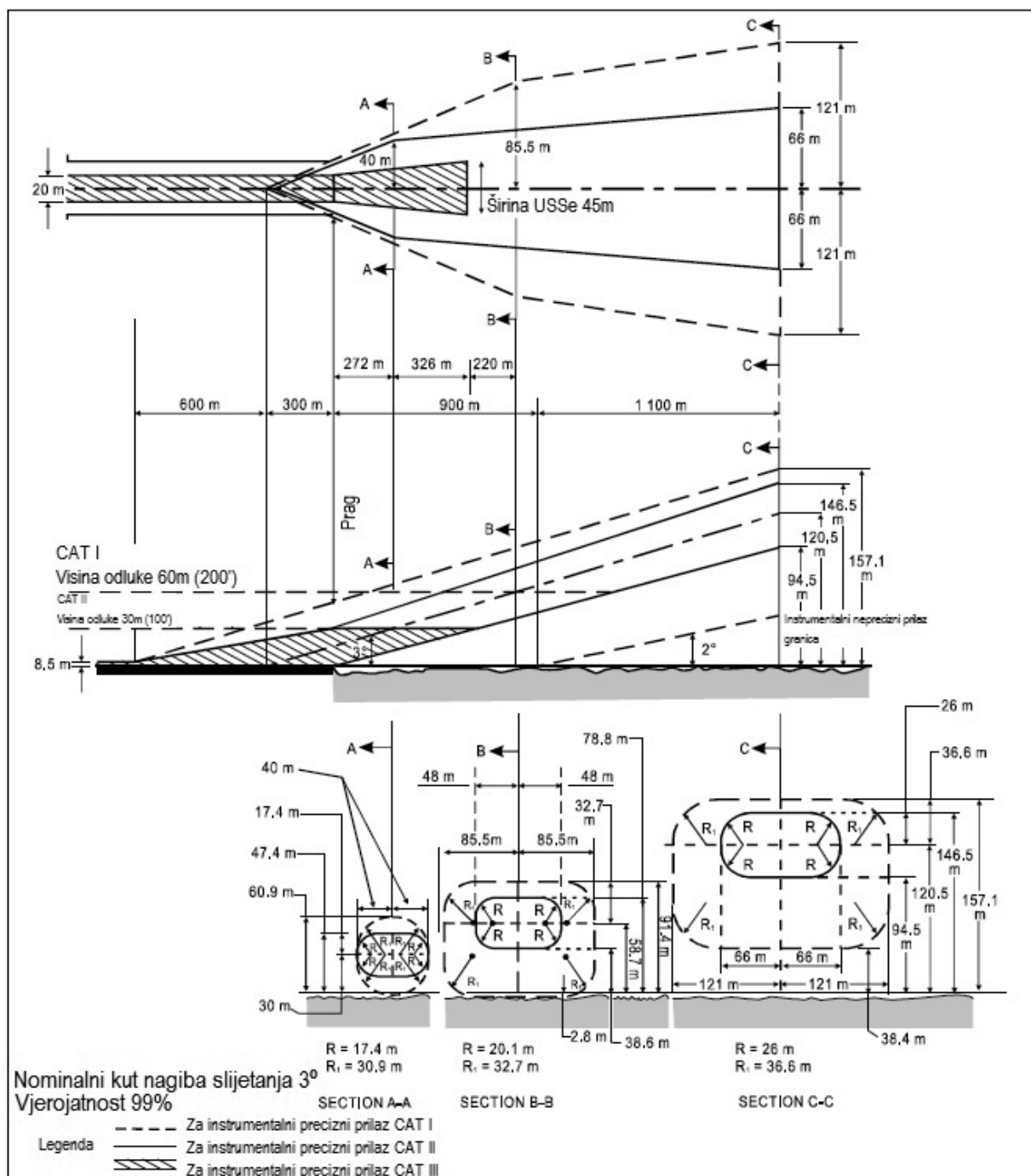
Slika A-5. Dijagrami putanje leta koji se moraju koristiti za projektiranje sustava rasvjete za uzletno-sletne staze sa CAT I, II i III
