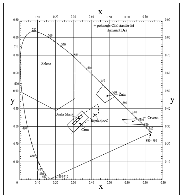
Slika A1-4. Boje svjetlićih ili transluminiranih (iznutra osvijetljenih) znakova i ploča
