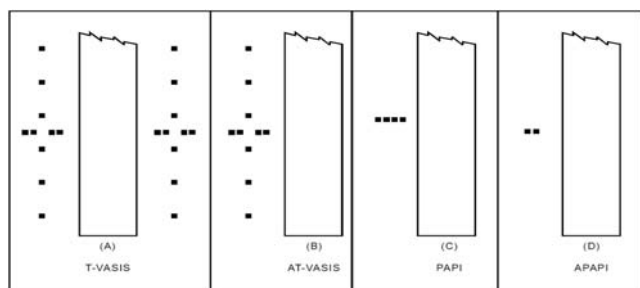
Slika 5-17. Sustavi svjetlosnih pokazivača nagiba prilaza
