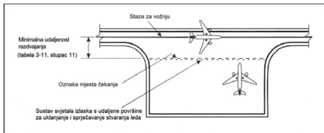
Slika 5-28. Tipična udaljena površina za uklanjanje i sprječavanje stvaranja leda
