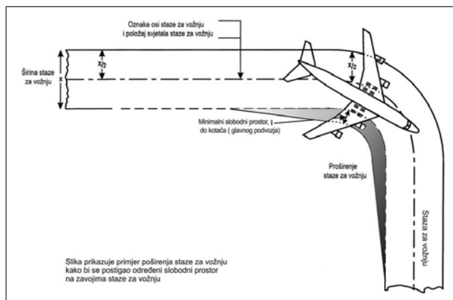
Slika 3-2. Zavoji na stazi za vožnju
