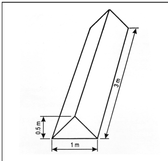
Slika 5-34. Označivač granice
