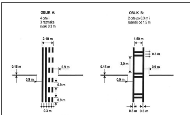
Slika 5.8. Oznake pozicije za čekanje
