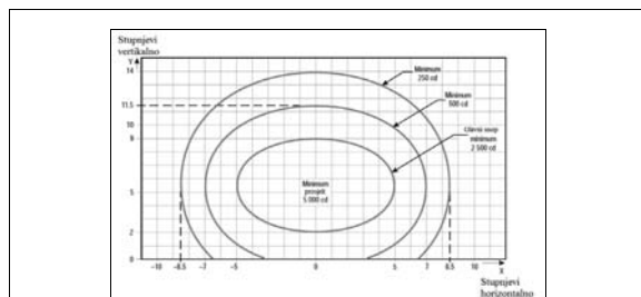
Slika A2-4. Dijagram izokandela za svjetlo praga krilne prečke (zeleno svjetlo)
