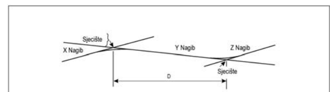
Slika A-2. Profil na središnjoj crti uzletno-sletne staze
