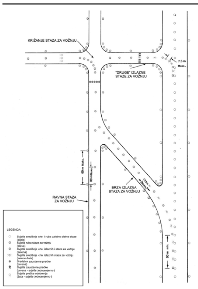
Slika 5-26 Sustavi svjetala staze za vožnju
