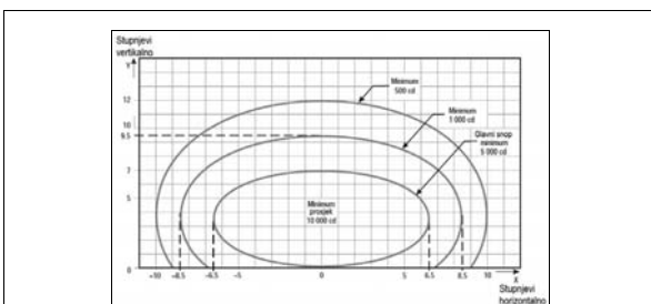
Slika A2.-9. Dijagram izokandela za rubno svjetlo uzletno-sletne staze širine 45 m (bijelo svjetlo)
