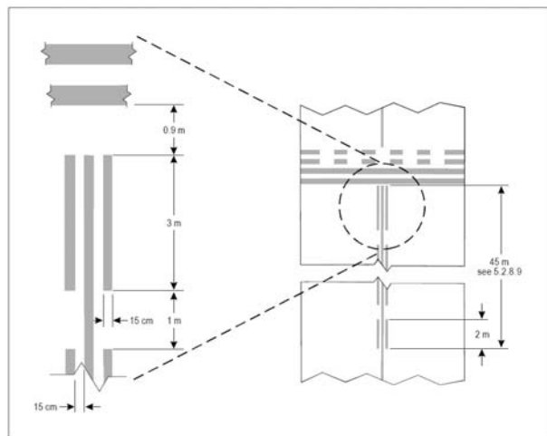
Slika 5-7. Dodatno istaknuta oznaka središnje crte staze za vožnju
