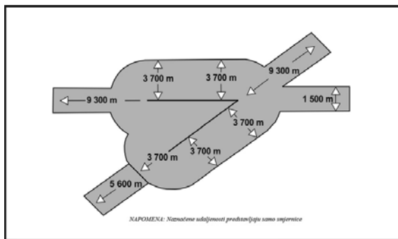
Slika 5-13. Područje letenja bez utjecaja laserskog zračenja na primjeru dviju uzletno-sletnih staza
