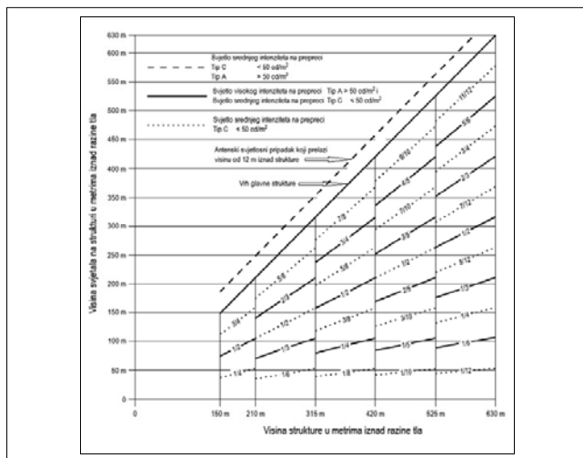
Slika A6-6. Sustav bijelih treptajućih svjetala visokog intenziteta, tipa A, na prepreci
