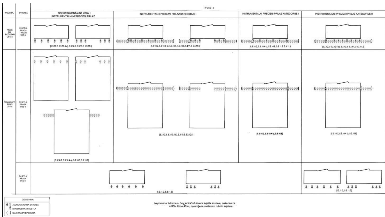
Slika 5-23. Raspored jediničnih izvora sustava svjetala praga uzletno-sletne staze i svjetala kraja uzletno-sletne staze
