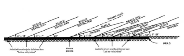
Slika 5-19. Snopovi svjetla koje odašilju jedinični izvori sustava T-VASIS i AT-VASIS, te podešavanje nagiba prilaza
