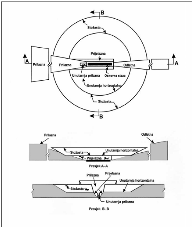
Slika 4-1 Površine ograničenja prepreka
