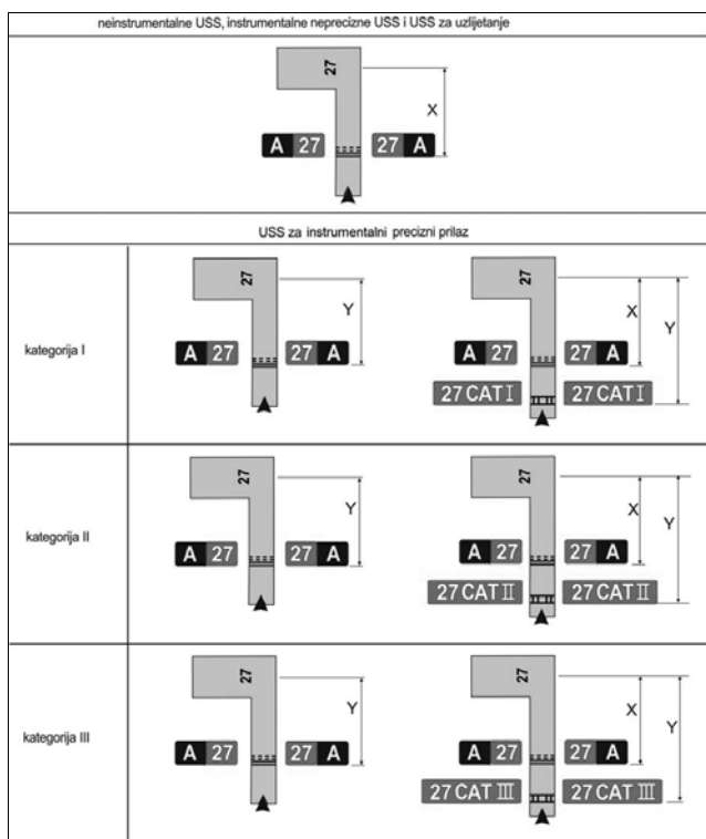
Udaljenost X mora biti u skladu s tabelom 3-2. Udaljenost Y definirana je rubom kritičnog/osjetljivog područja sustava ILS/MLS
