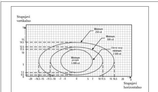
Slika A2-1. Dijagram izokandela za svjetlo proizvedene središnje crte sustava prilazne rasvjete i poprečne prečke (bijelo svjetlo)
