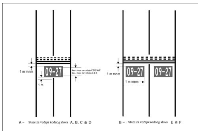
Slika 5-11. Oznake naredbi
