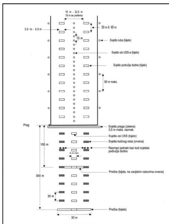
Slika 5-15. Unutarnjih 300 m svjetala prilaza i svjetala uzletno-sletne staze kod uzletno-sletnih staza za precizni prilaz kategorije II ili III
