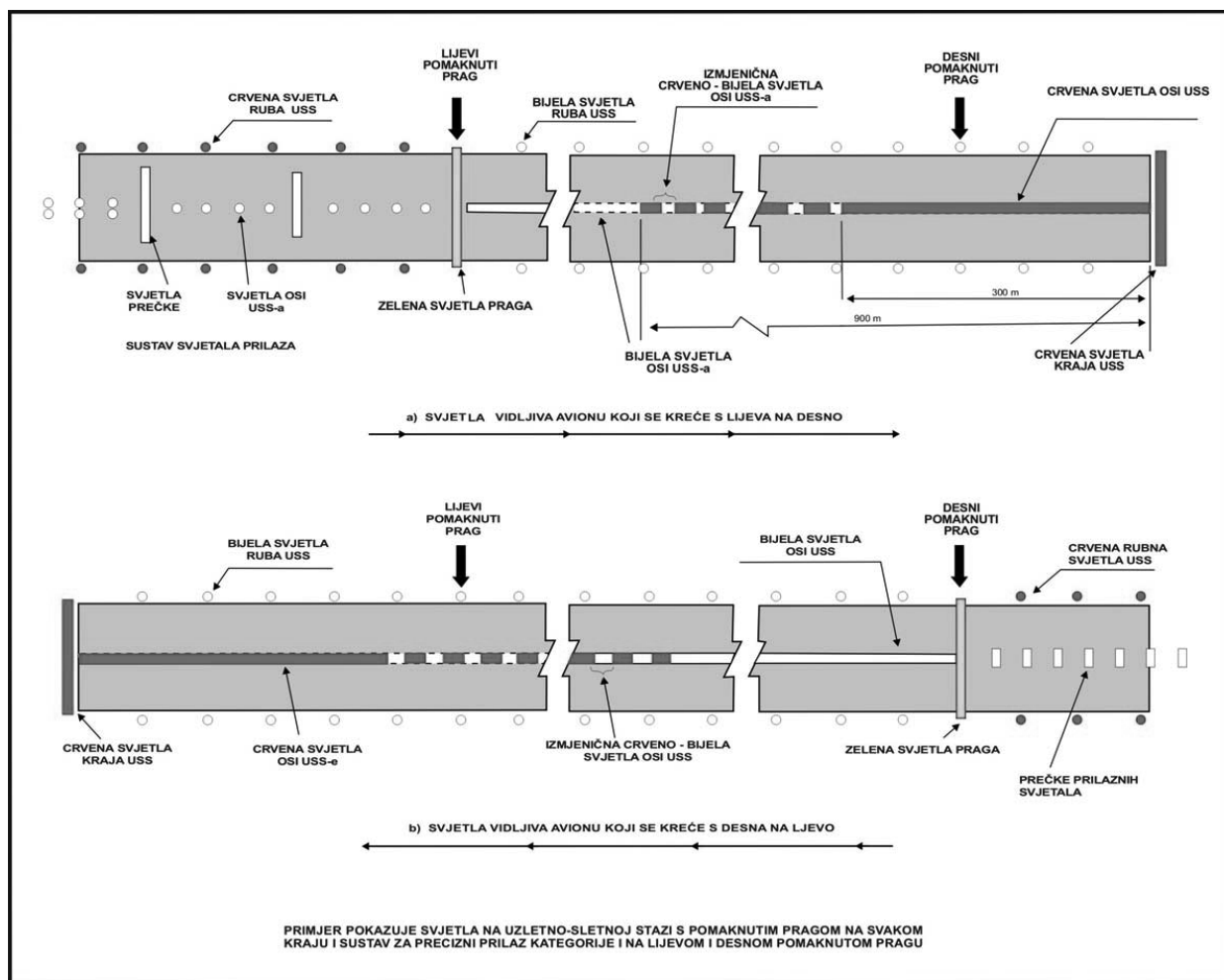
Slika 5-24. Primjer prilazne rasvjete i rasvjete uzletno-sletne staze s pomaknutim pragom
