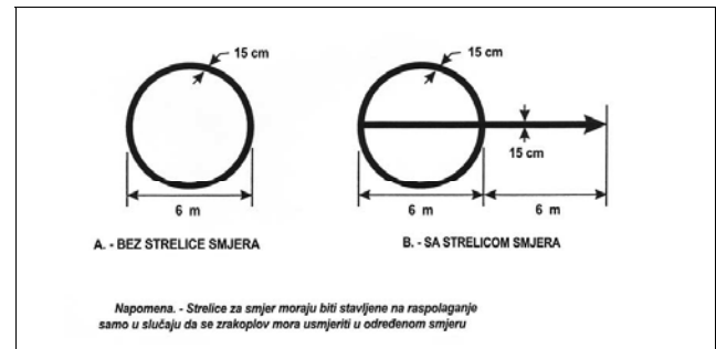
Slika 5-9. Oznaka VOR kontrolne točke aerodroma
