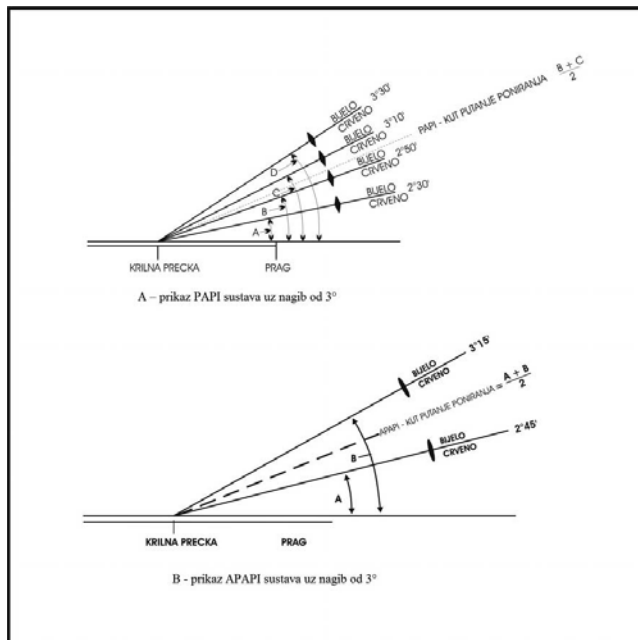
Slika 5-21 Nagib prilaza definiran za sustave PAPI i APAPI
