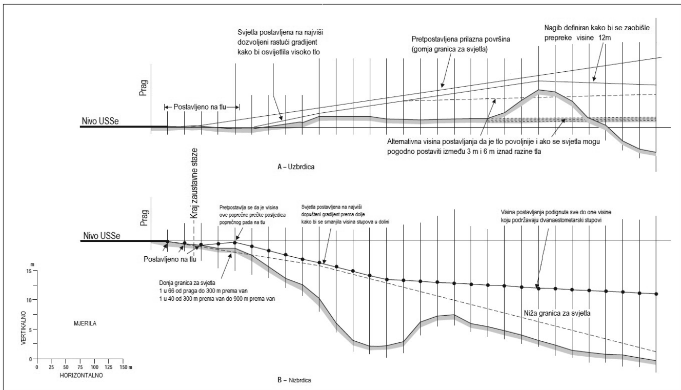
Slika A-8. Okomito dozvoljeno odstupanje instaliranja
