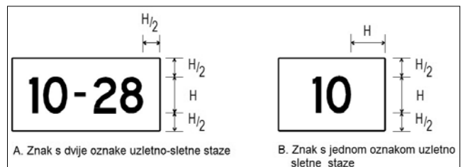
Slika A4.-3. Dimenzije znakova
