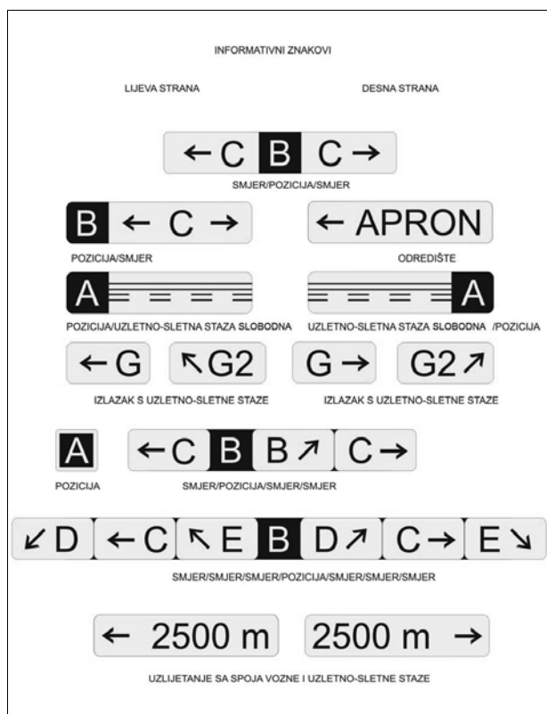
Slika 5-31. Informativni znakovi
