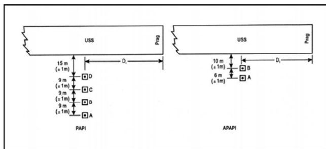
Slika 5-20. Tipična krilna prečka PAPI sustava/Tipična krilna prečka APAPI sustava
