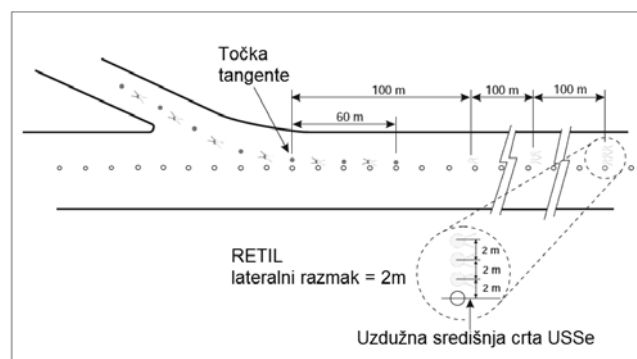
Slika 5-25. Svjetlosni pokazivači brzih izlaznih staza za vožnju
