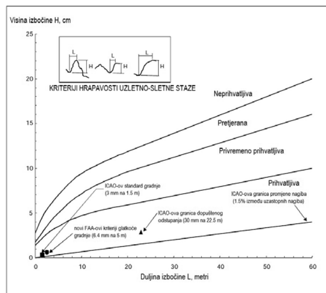
Slika A-3. Usporedba kriterija hrapavosti
