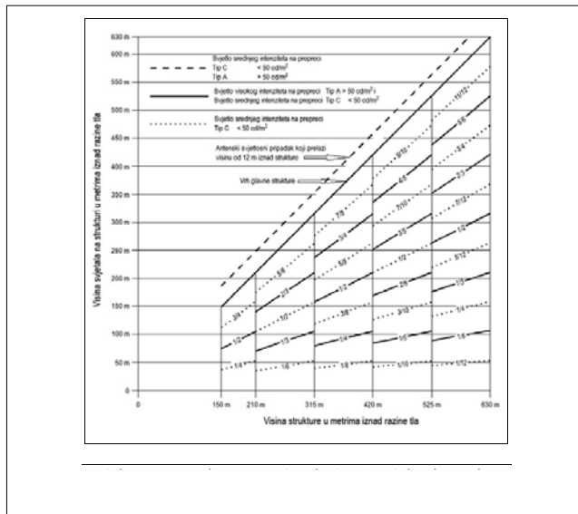
Slika A6-8. Dualni sustav rasvjete prepreka visokog/srednjeg intenziteta, tipa A/tipa C
