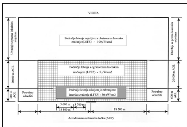
Slika 5-14. Zaštićena područja letenja s najvišim dozvoljenim vrijednostima isijavanja vidljivih laserskih zraka (AGL = iznad razine tla)
