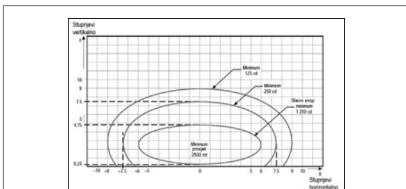
Slika A2.-7. Dijagram izokandela za svjetlo središnje crte USSe longitudinalnog razmaka 15 m (bijelo svjetlo) i kratkog svjetla pokazatelja izlazne staze za vožnju (žuto svjetlo)
