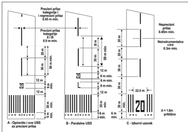
Slika 5-2. Oznake uzletno-sletne staze, središnje crte i praga
