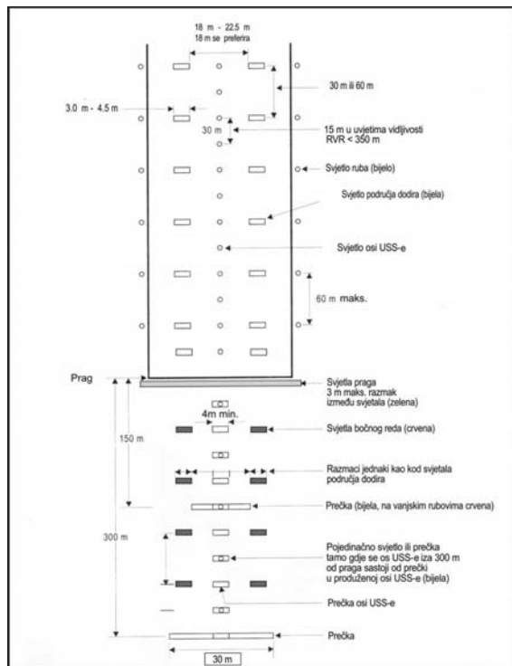
Slika 5-16. Unutarnjih 300 m sustava prilazne rasvjete i sustava rasvjete uzletno-sletne staze za instrumentalni precizni prilaz kategorije II ili III, ukoliko operator aerodroma osigura ispravnost sustava prilazne rasvjete definiran u članku 189. stavku 8. ovoga Pravilnika
