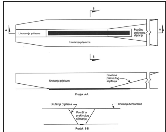
Slika 4-2 Površine ograničenja prepreka: unutarnja prilazna, unutarnja prijelazna i površina prekinutog slijetanja
