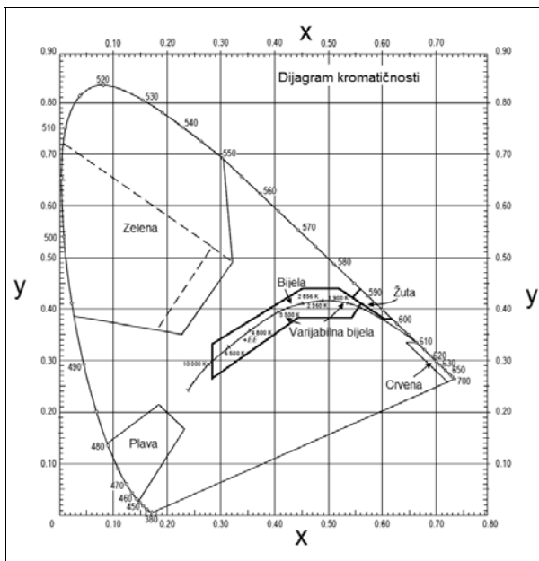
Slika A1-1. Boje za aeronautička svjetla na tlu
