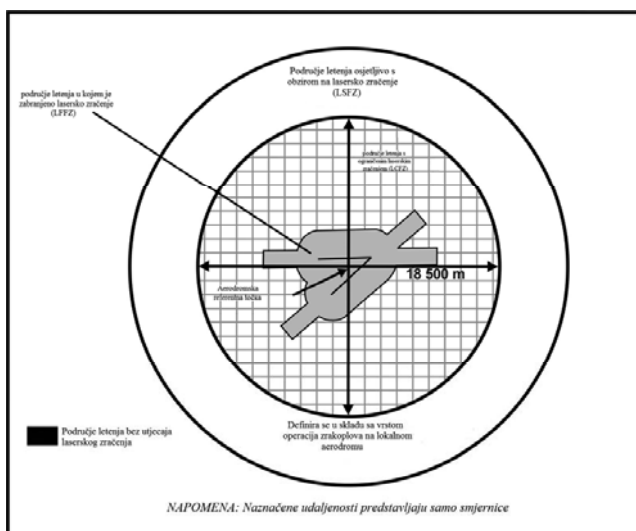
Slika 5-12. Područje letenja bez utjecaja laserskog zračenja
