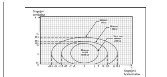
Slika A2-3. Dijagram izokandela za svjetlo praga (zeleno svjetlo)
