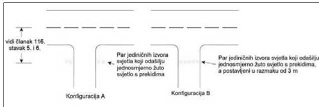
Slika 5-29. Sustav sigurnosnih svjetala uzletno-sletne staze
