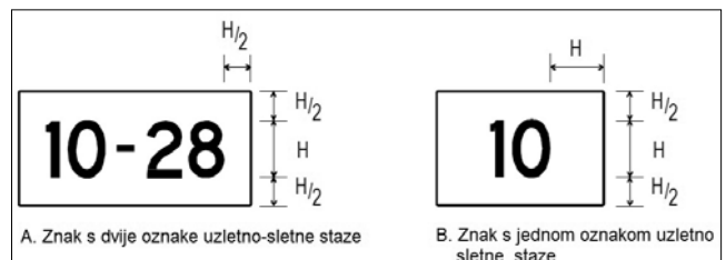
Slika A4.-3. Dimenzije znakova
