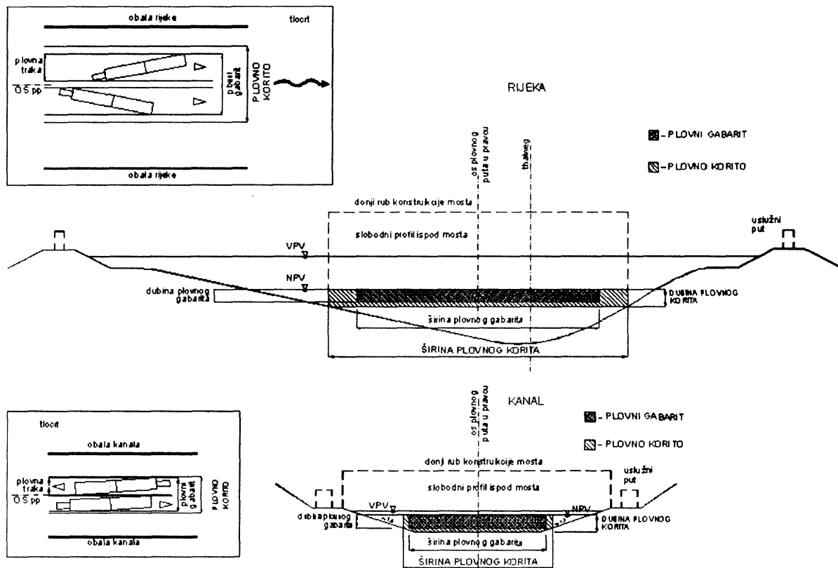
SI.3 Definicijska skica za tipski poprečni presjek plovnoг puta u pravcu na rijeci i kanalu
