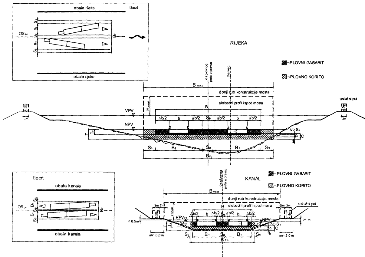
SI.4 Definicijske skice širine i dubine dvosmjernog plovnoг puta u pravcu na rijeci za mjerodavan slučaj pretjecanja te na kanalu za mjerodavan slučaj mimoilaženja
